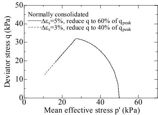
Fig. 6 p' - q plots (NC)
