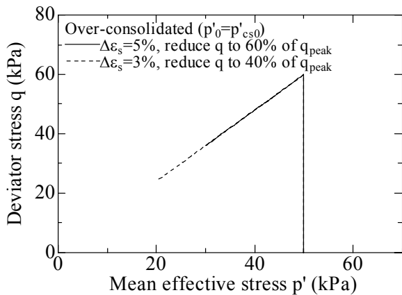
Fig. 8 p' - q plots (OC-1)
