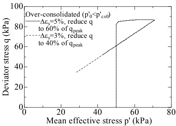
Fig. 10 p' - q plots (OC-2)
